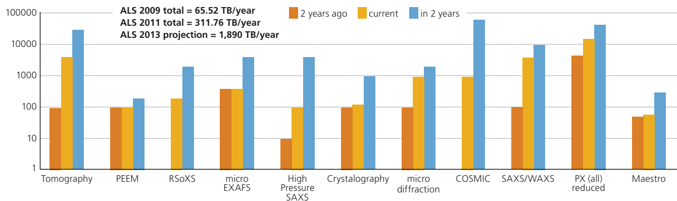
// Figure 4. Growing ALS data rates.
